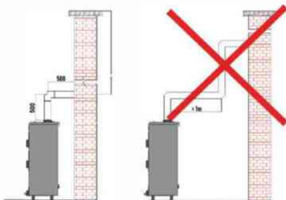
Figura nr. 1 - Racordarea corectă și incorectă a coșului de fum
